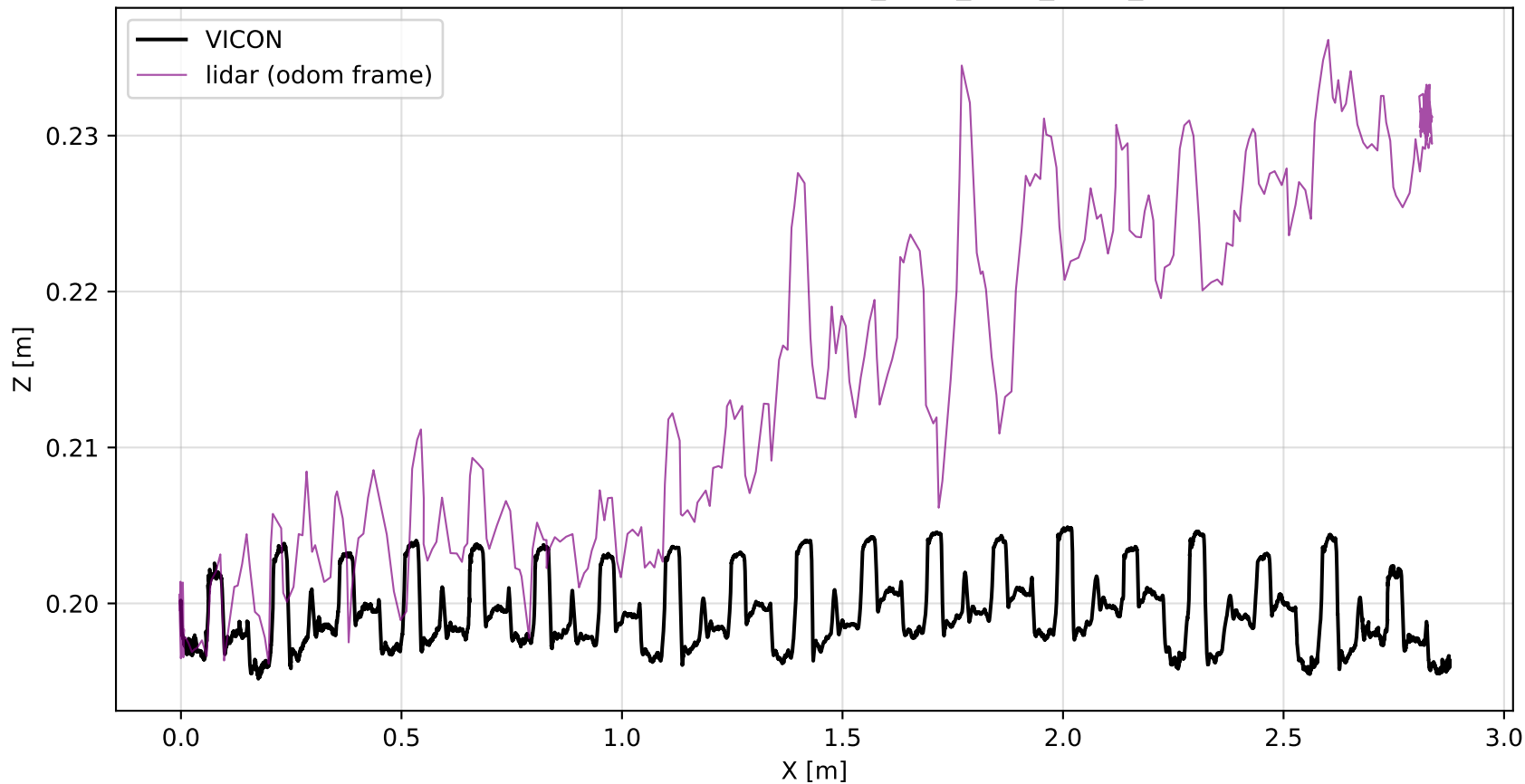
LiDAR XZ Trajectory — FLAT_WLW_NEW_REAL_3
