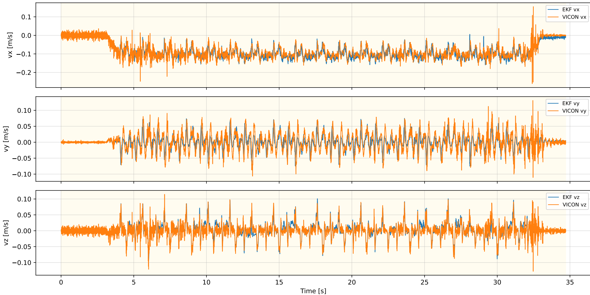
Inner EKF Velocity — FLAT_WLW_NEW_REAL_4
