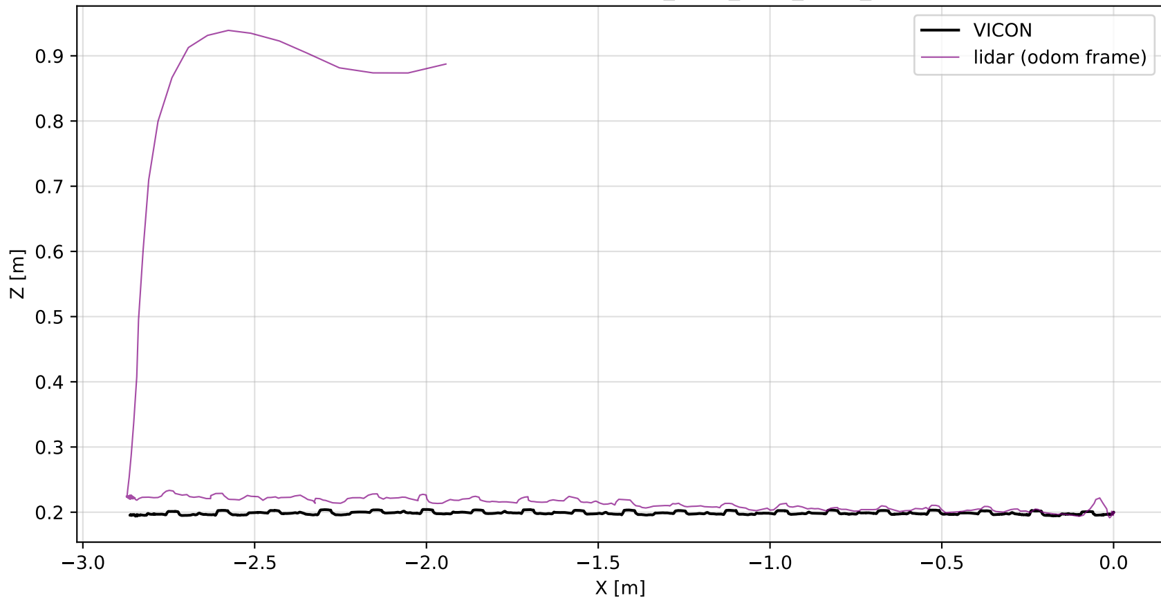
LiDAR XZ Trajectory — FLAT_WLW_NEW_REAL_4
