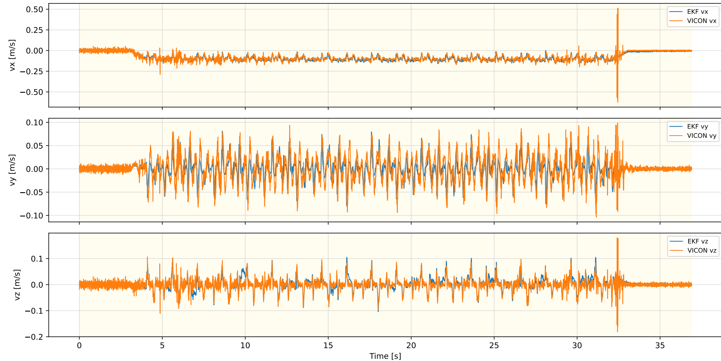
Inner EKF Velocity — FLAT_WLW_NEW_REAL_5
