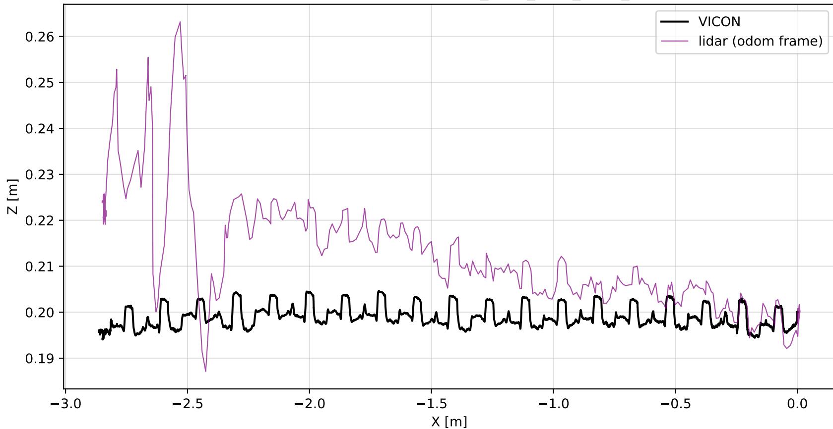
LiDAR XZ Trajectory — FLAT_WLW_NEW_REAL_5
