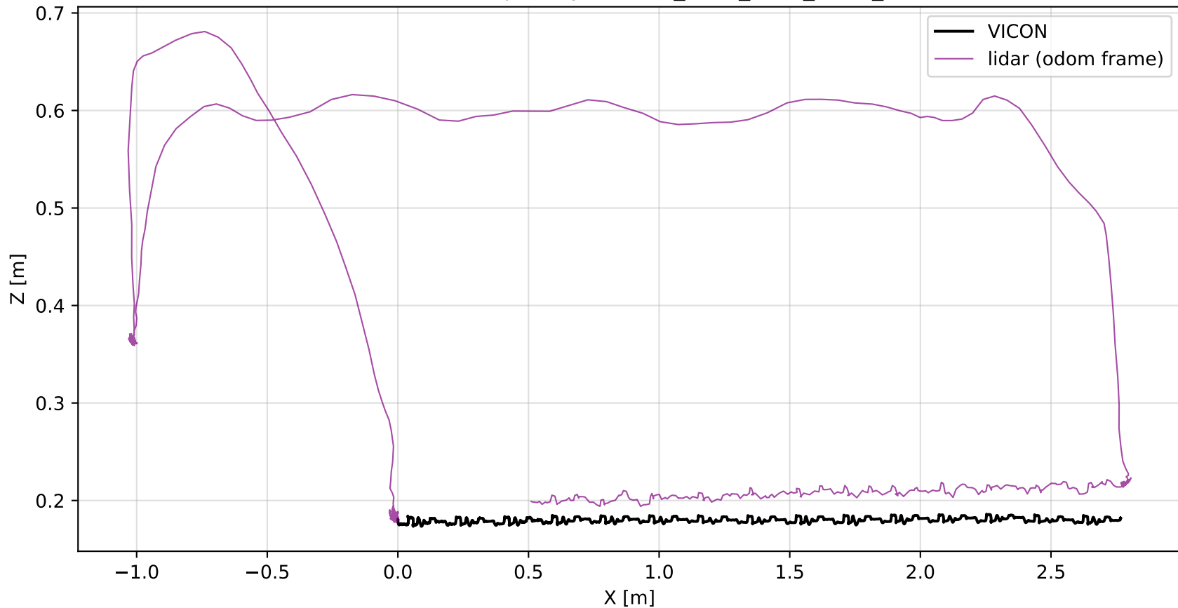
LiDAR XZ Trajectory — FLAT_Walk_NEW_REAL_1
