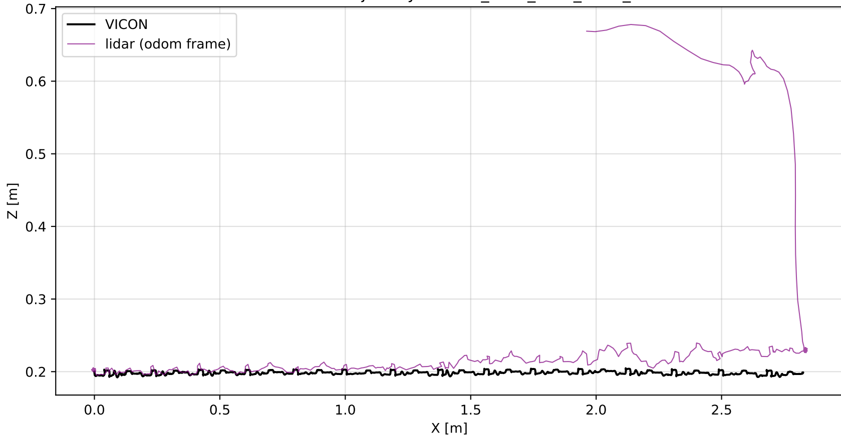
LiDAR XZ Trajectory — FLAT_Walk_NEW_REAL_6
