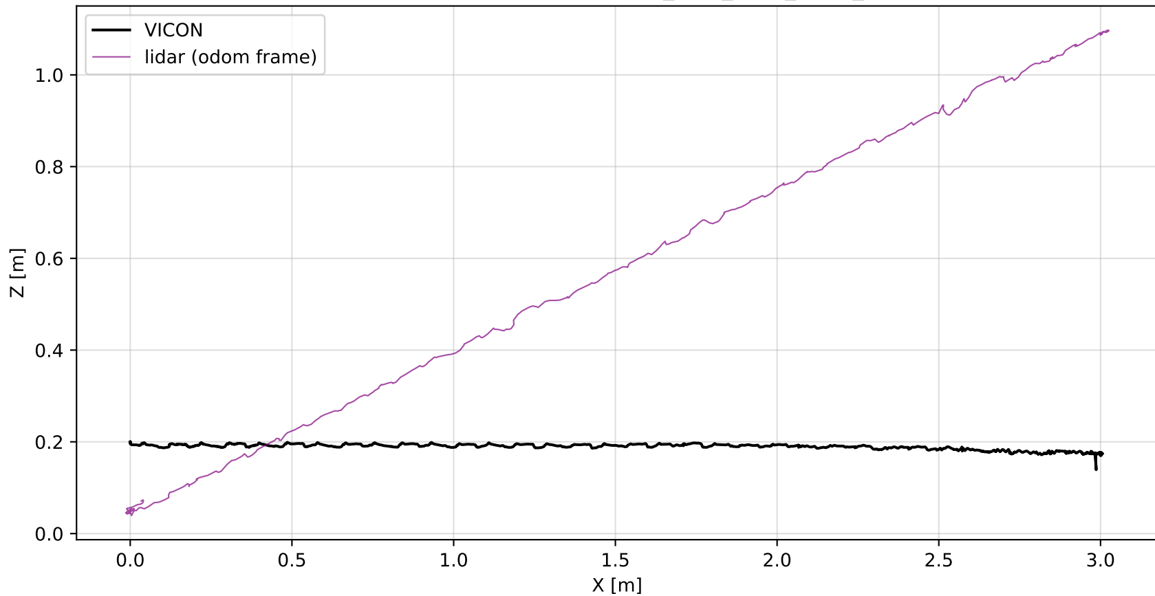
LiDAR XZ Trajectory — FLAT_MPC_NEW_REAL_4
