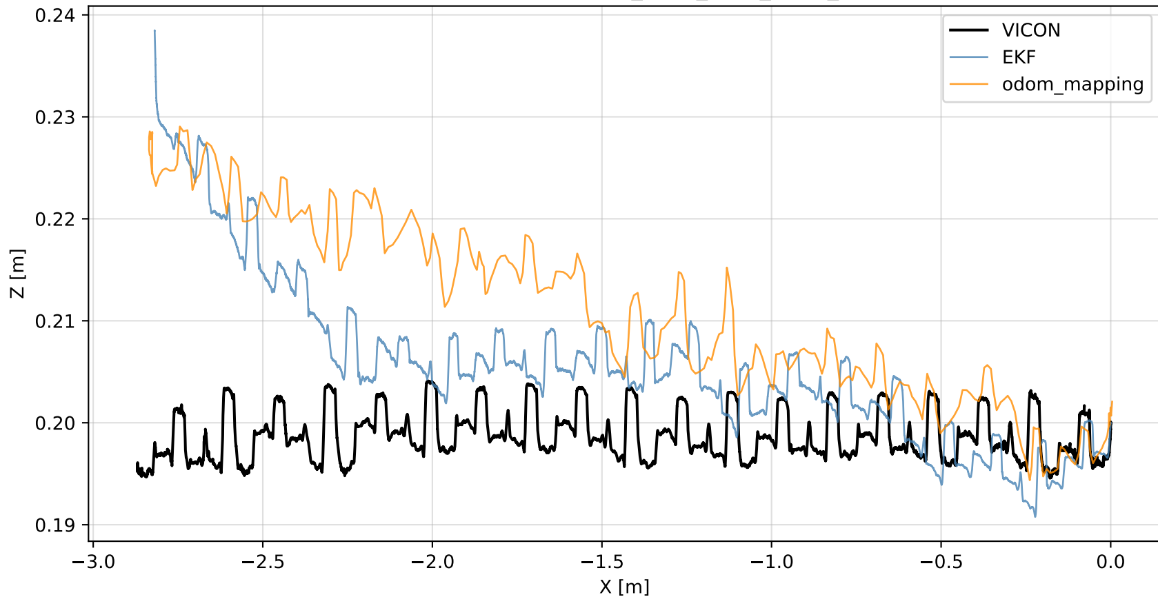
XZ Trajectory — FLAT_WLW_NEW_REAL_2
