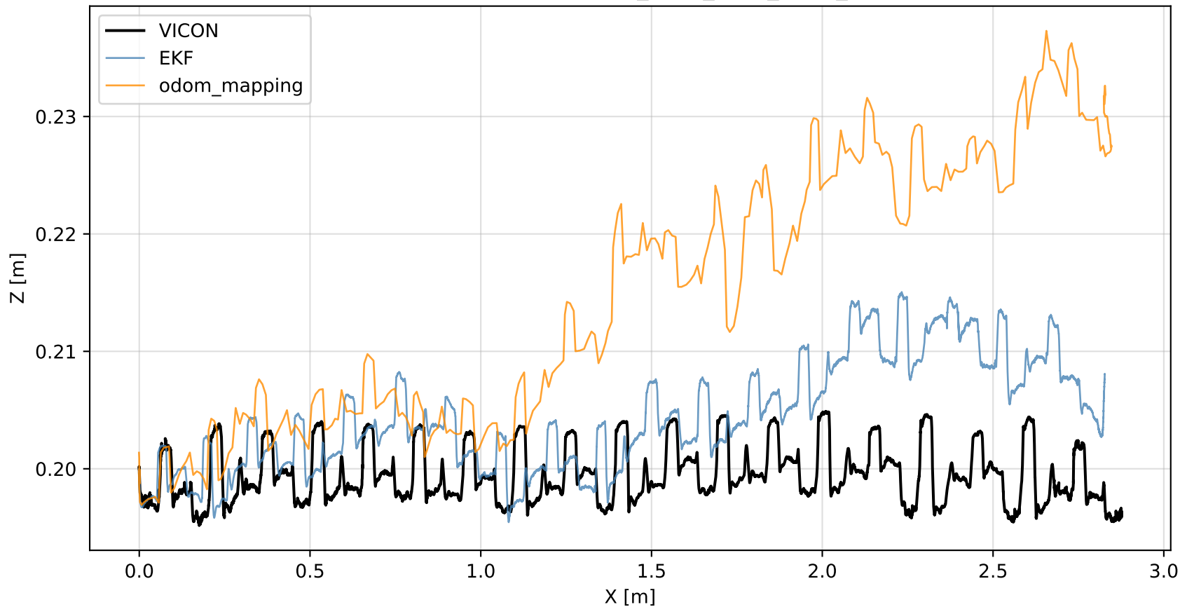
XZ Trajectory — FLAT_WLW_NEW_REAL_3
