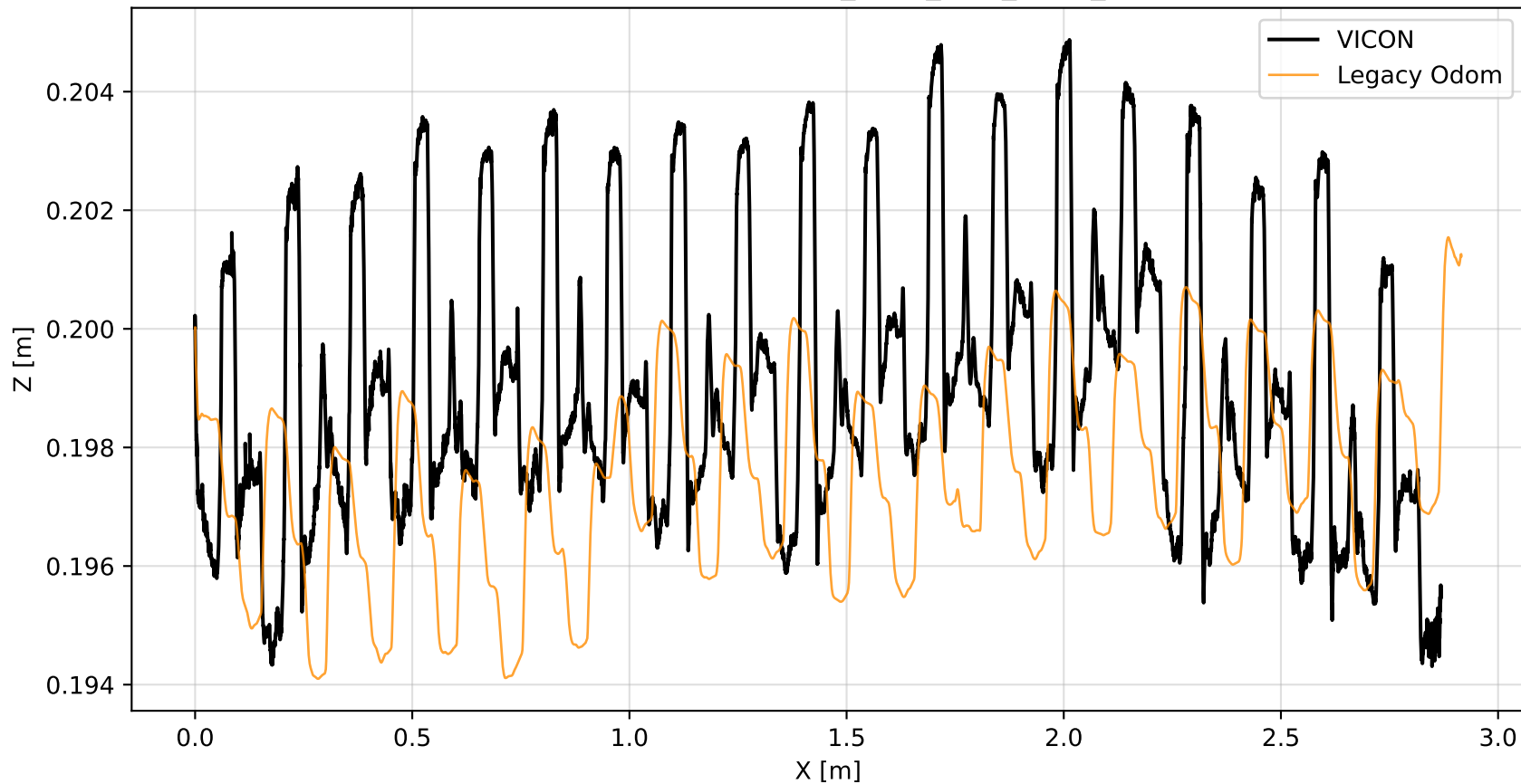
XZ Trajectory — FLAT_WLW_OLD_REAL_2
