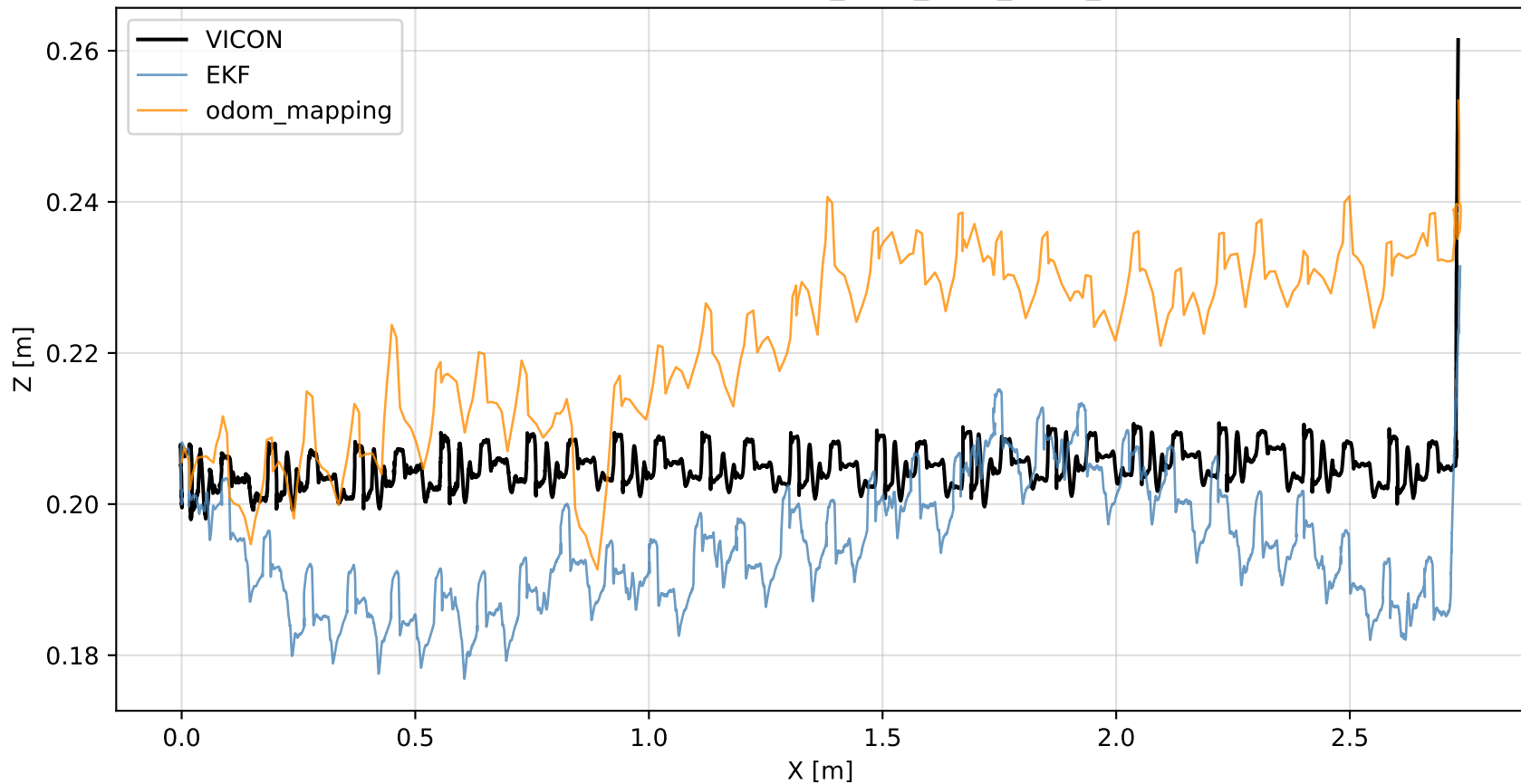
XZ Trajectory — FLAT_Walk_NEW_REAL_3
