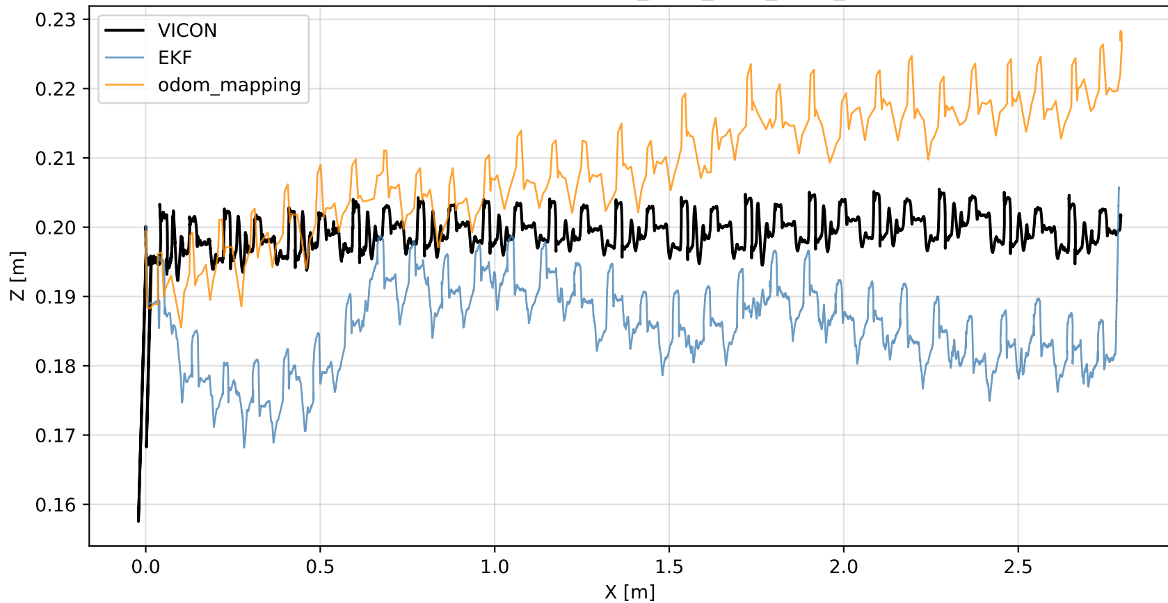
XZ Trajectory — FLAT_Walk_NEW_REAL_4
