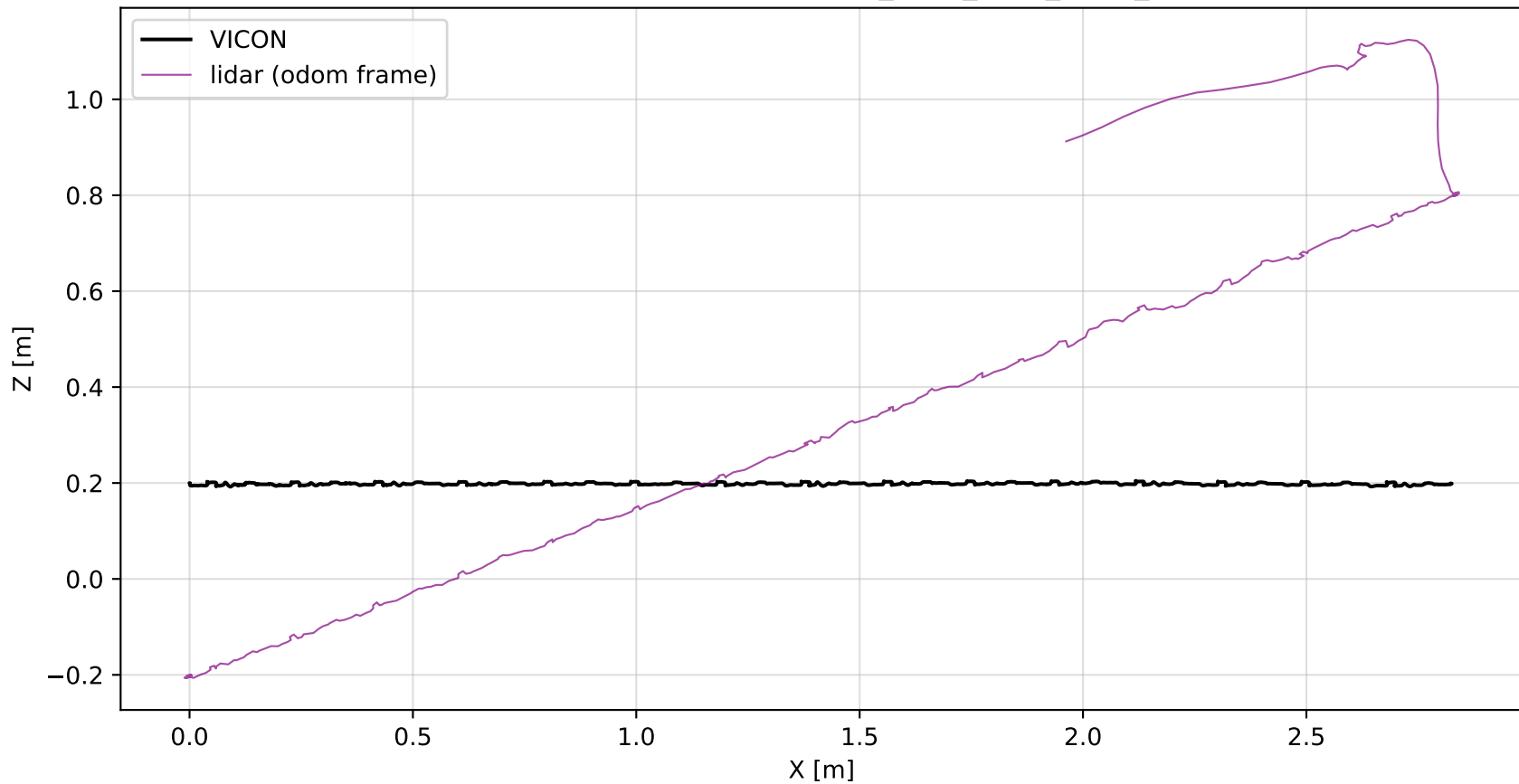
LiDAR XZ Trajectory — FLAT_Walk_NEW_REAL_6
