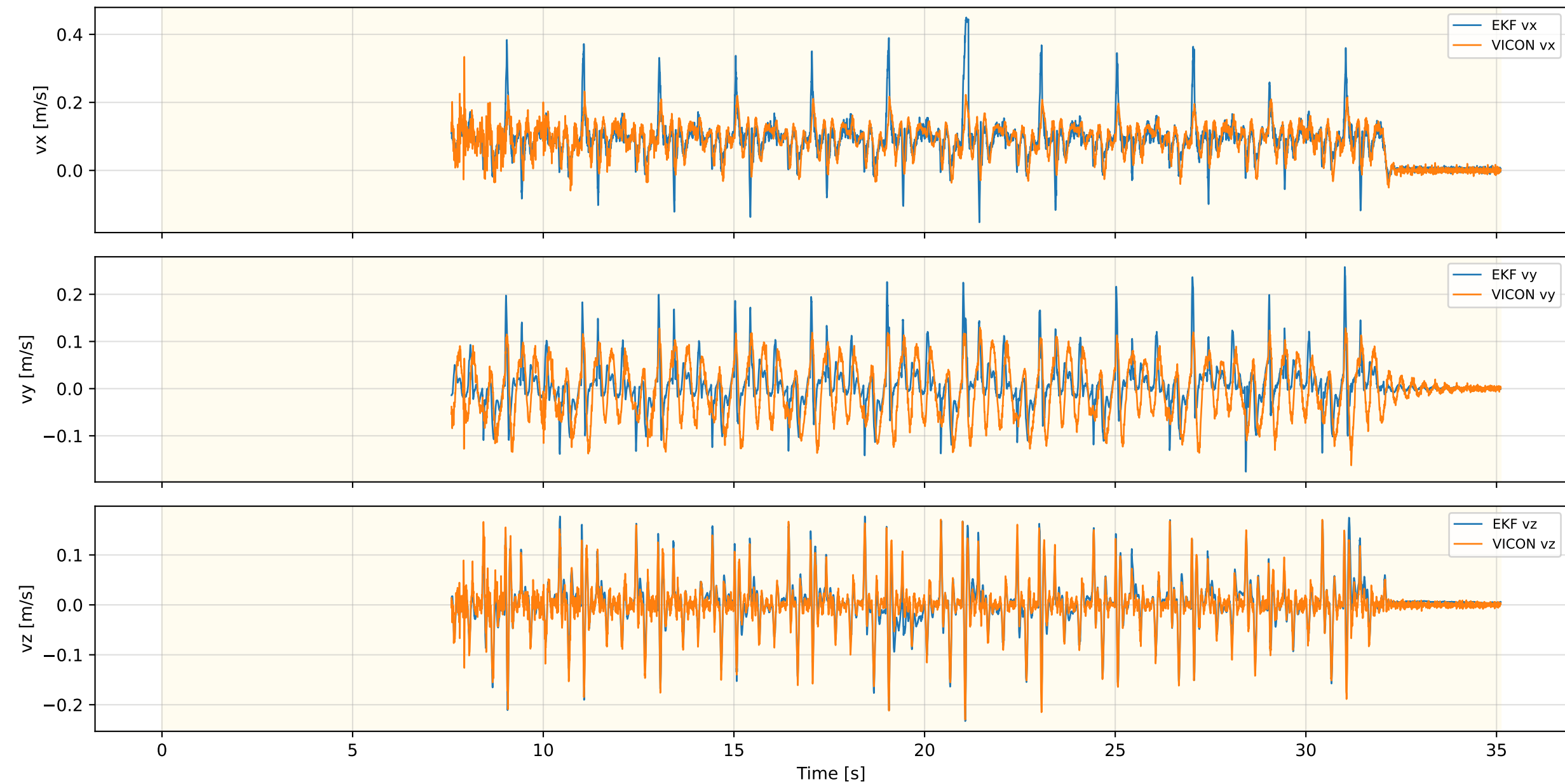
Inner EKF Velocity — FLAT_Walk_NEW_REAL_1
