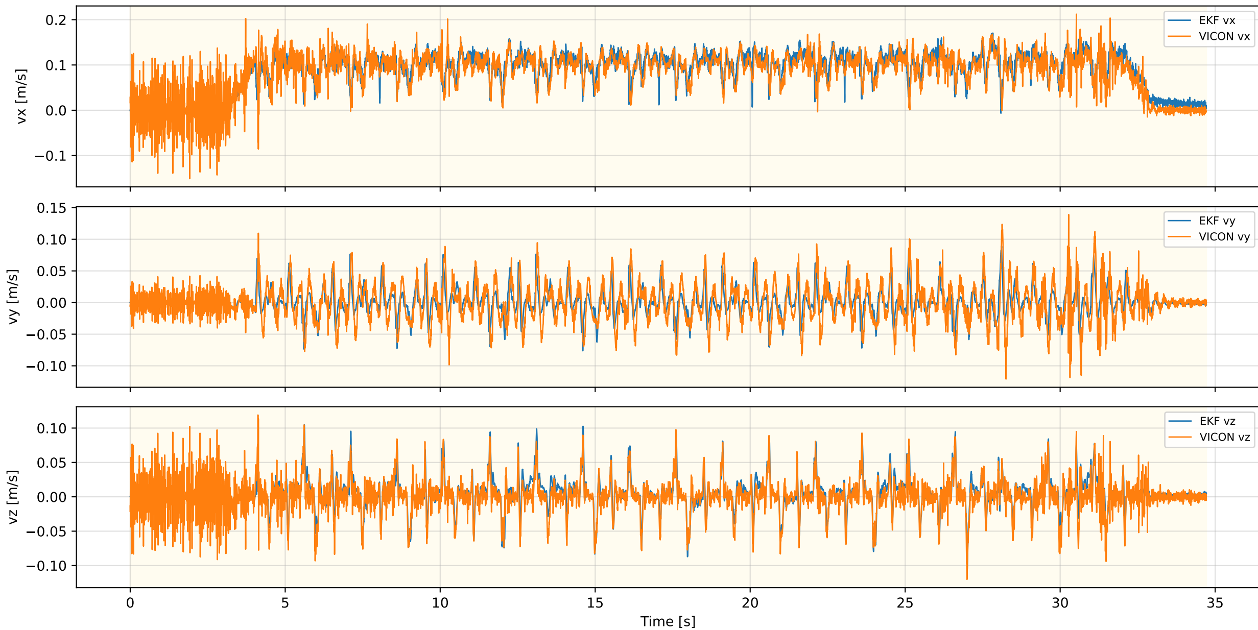
Inner EKF Velocity — FLAT_WLW_NEW_REAL_1
