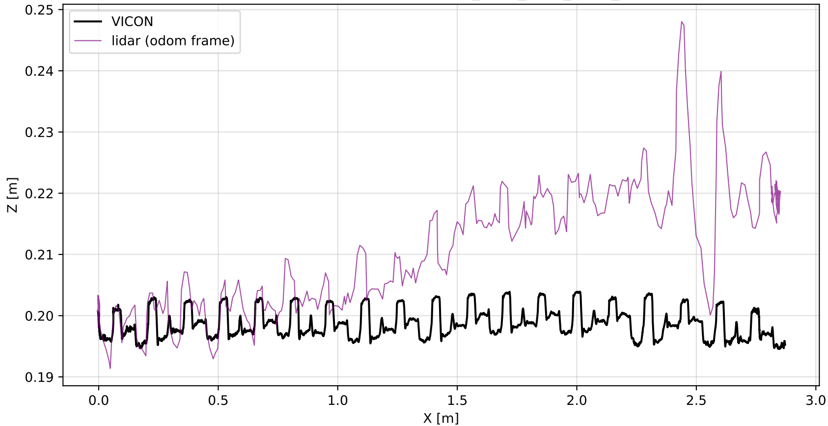
LiDAR XZ Trajectory — FLAT_WLW_NEW_REAL_1
