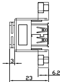
CN1 U3_A9F_DUAL 9 PIN*2 5XPL-227-G PVC 35P 黑色外模
