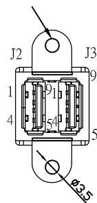
M3螺母(5XSC-065) 後塞緊配
