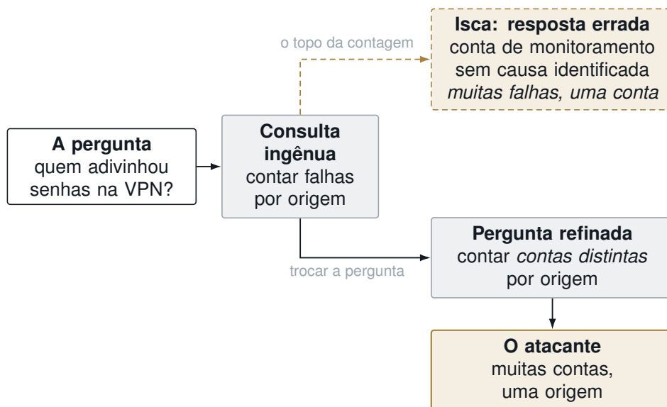
Figura 1.2. A anatomia de uma isca, no formato dos três estudos de caso. A consulta mais óbvia tem uma resposta, e ela é uma rotina legítima. A caçada só avança quando a pergunta muda de quanto para quantos diferentes .
