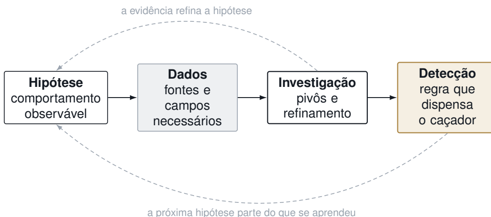
Figura 1.1. O ciclo de caça seguido nos estudos de caso, núcleo comum aos modelos PEAK e TaHiTI.
