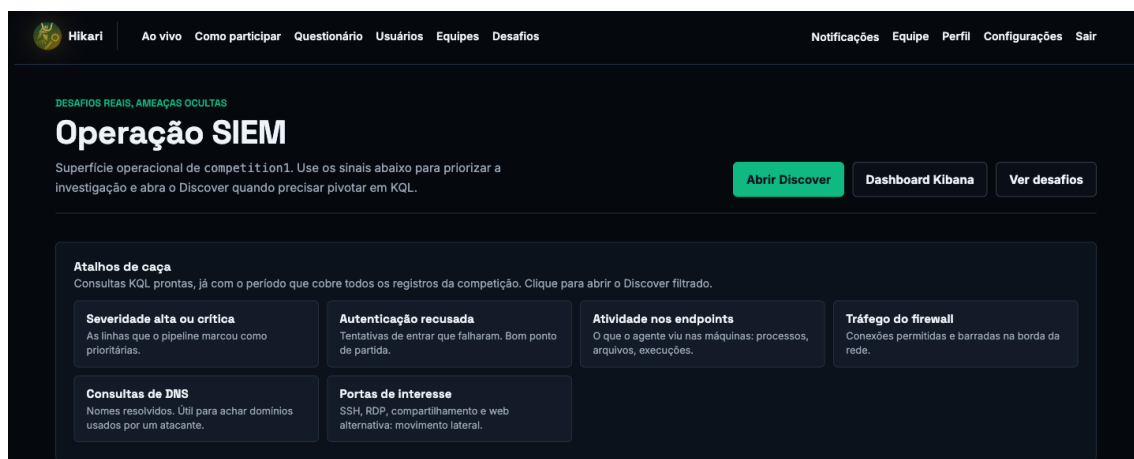
Figura 1.4. A superfície do SIEM, com os atalhos de caça que abrem o Discover já filtrado. Os números do topo são da instalação usada para a figura, e não do cenário Aurora.
