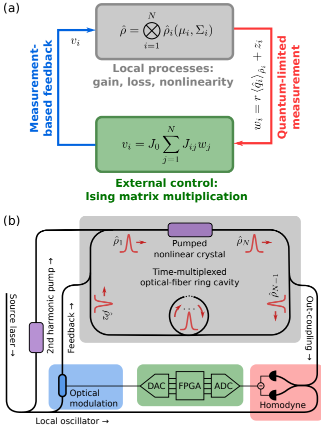
図1. 測定フィードバック型コヒーレントイジングマシン (MFB-CIM) の概略。(a) 抽象的には、MFB-CIMはN個の光学モードからなる系（灰色の枠）であり、各モードの状態 \hat{\rho}_i は平均ベクトル \mu_i と共分散行列 \Sigma_i で特徴付けられる。各モードは光利得・損失・非線形性の作用を受ける。系を弱測定で調べることで、正規分布（ガウス分布）に従う量子雑音 z_i を伴う、同相成分 q_i の推定値 w_i を得る。この推定値を外部制御器（緑色の枠）が処理し、指定されたイジング問題の行列 J_{ij} に基づくフィードバック信号 v_i を生成する。こうしてループを閉じると、イジング結合が系のダイナミクスに組み込まれる。(b) 時間多重方式[7, 8]によるMFB-CIMの光学構成。光パルス \rho_i が共振器内を循環し、励起された非線形結晶が利得と非線形性を与え、さらに付加的な線形損失が存在する。出力結合器で各パルスの一部を取り出して平衡光ホモダイン測定を行い、電気信号 w_i を得る。FPGAはこの信号を処理してフィードバック v_i を生成する。局部発振光の強度・位相を変調して光信号に再符号化し、共振器へ再注入することでパルスを光学的に変位させ、ループを閉じる。
