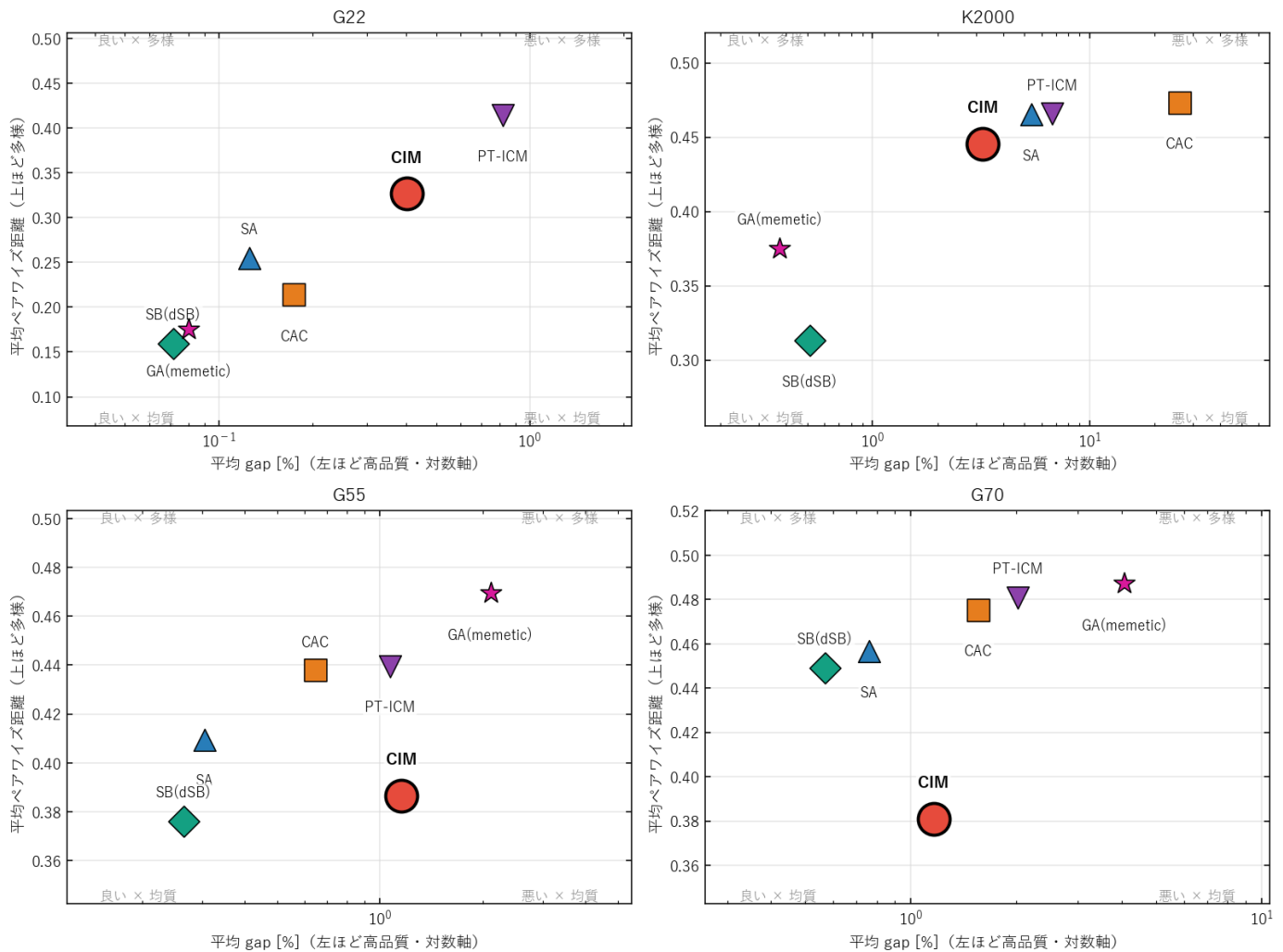
図1 手法の位置づけ：解は良いか／解はばらけるか
