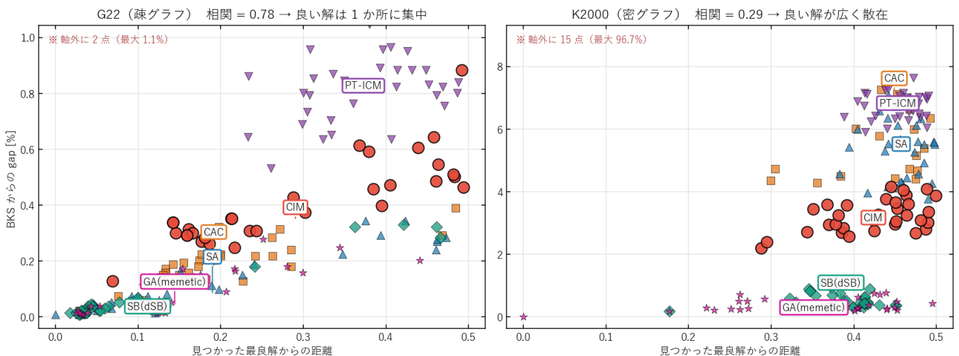
図5 良い解は1か所に集まるのか、あちこちに散るのか（枠は各手法の重心）
