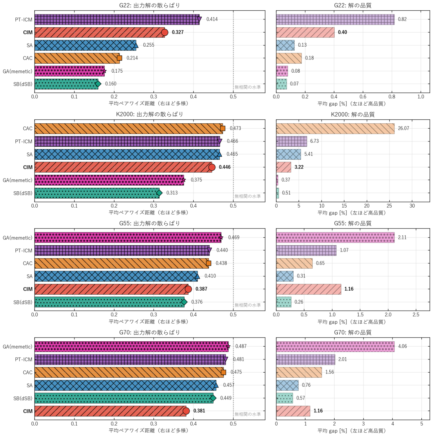
図2 同じ実時間で 32 回解いたときの「散らばり」と「良さ」
