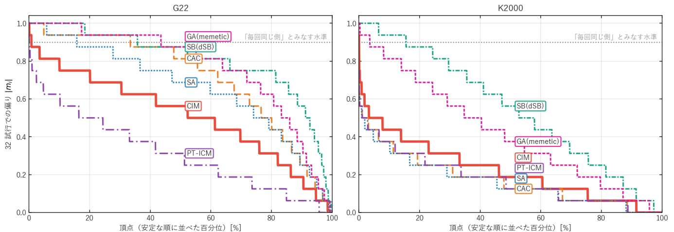
図3 どれだけの頂点が「毎回同じ側」に決まるか（曲線が高いほど骨格が太い）
