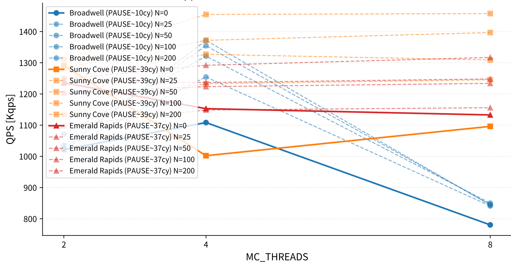
Approach A: QPS vs スレッド数 (固定N)
