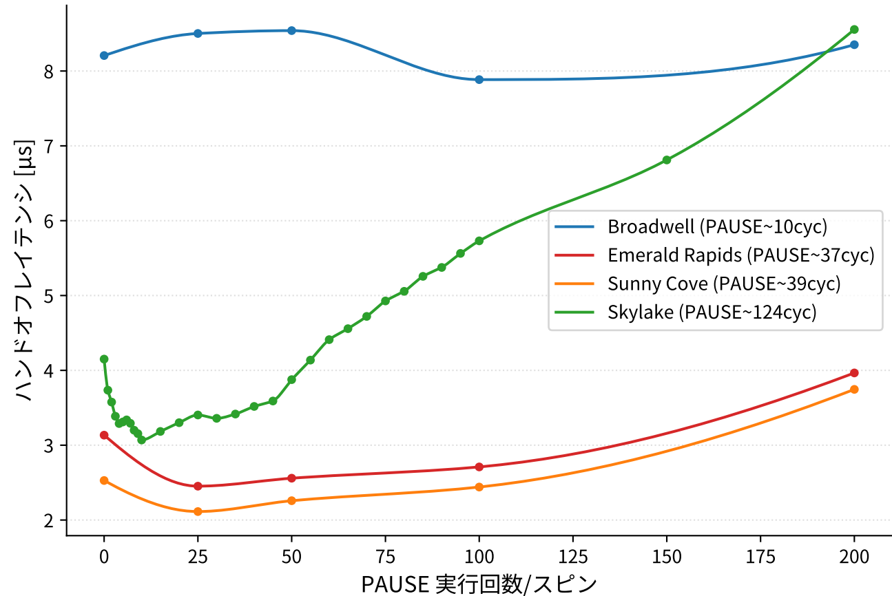
p99 ハンドオフレイテンシ
