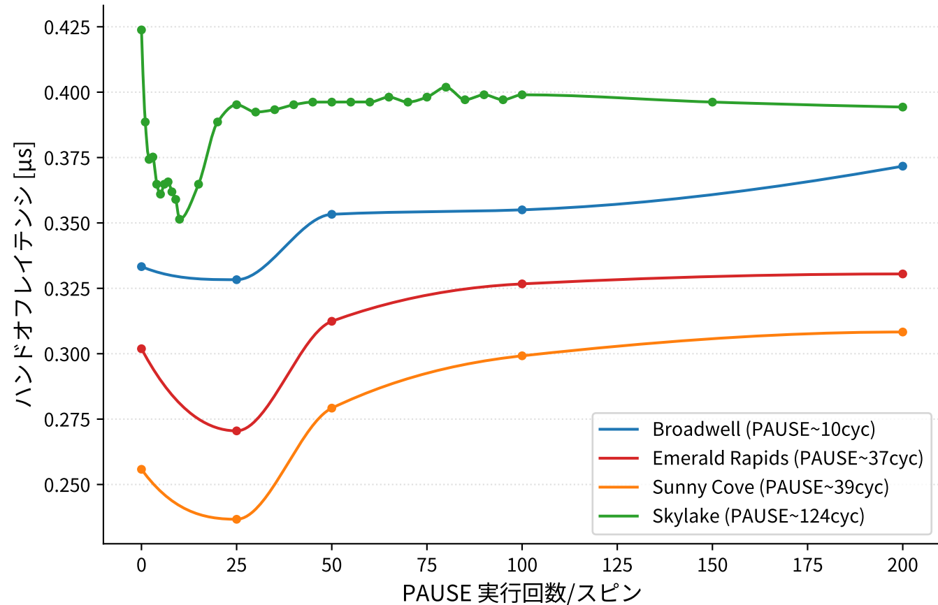
p50 ハンドオフレイテンシ
