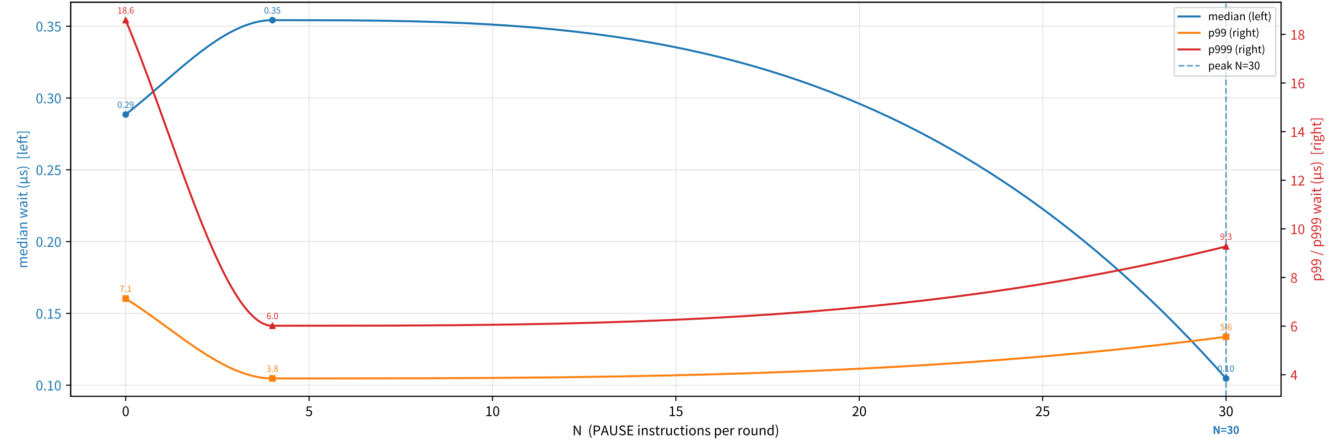
Skylake ann (Silver 4110, PAUSE~124cy) / TSC 2100 MHz
