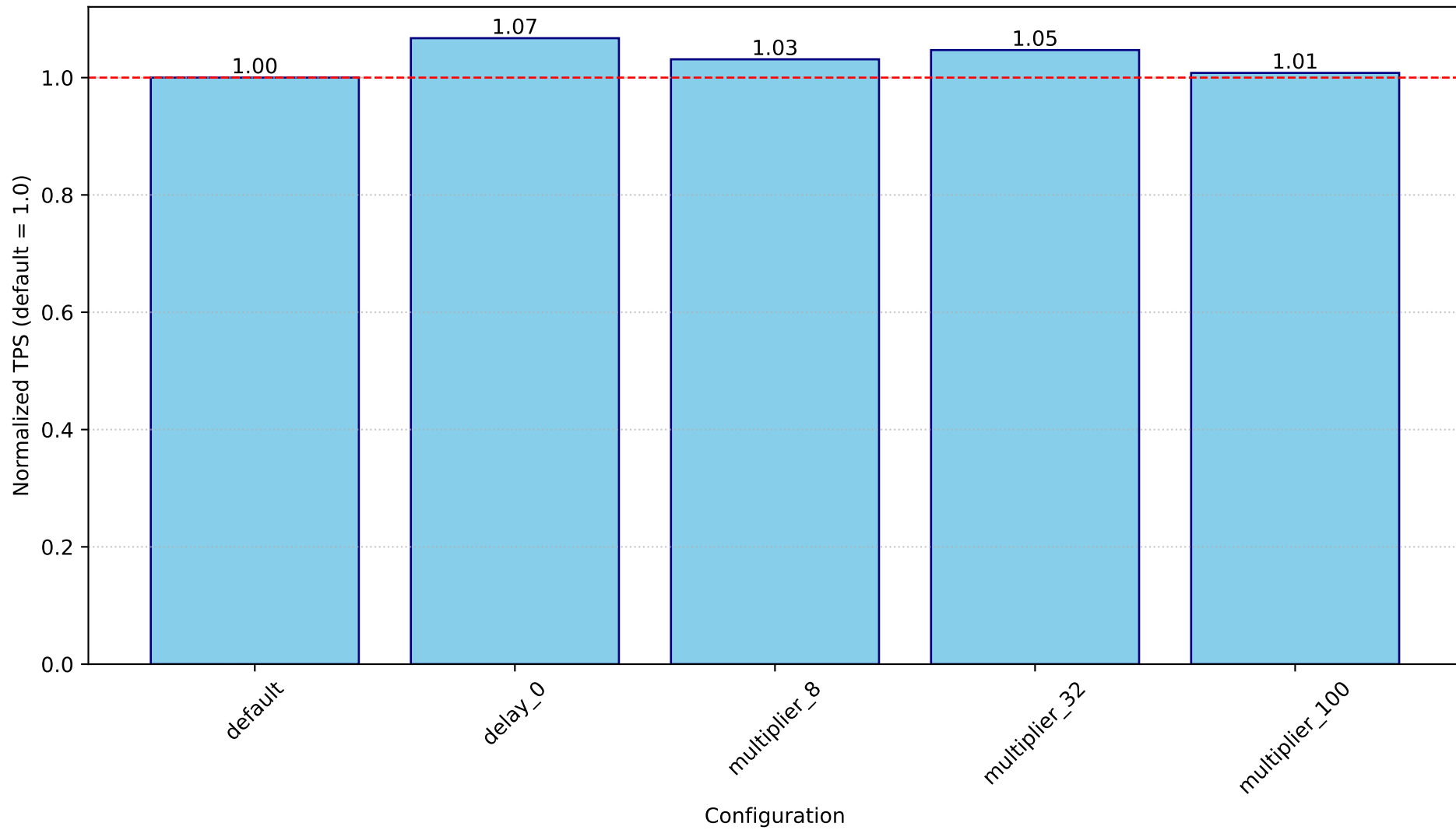
ann-skylake
