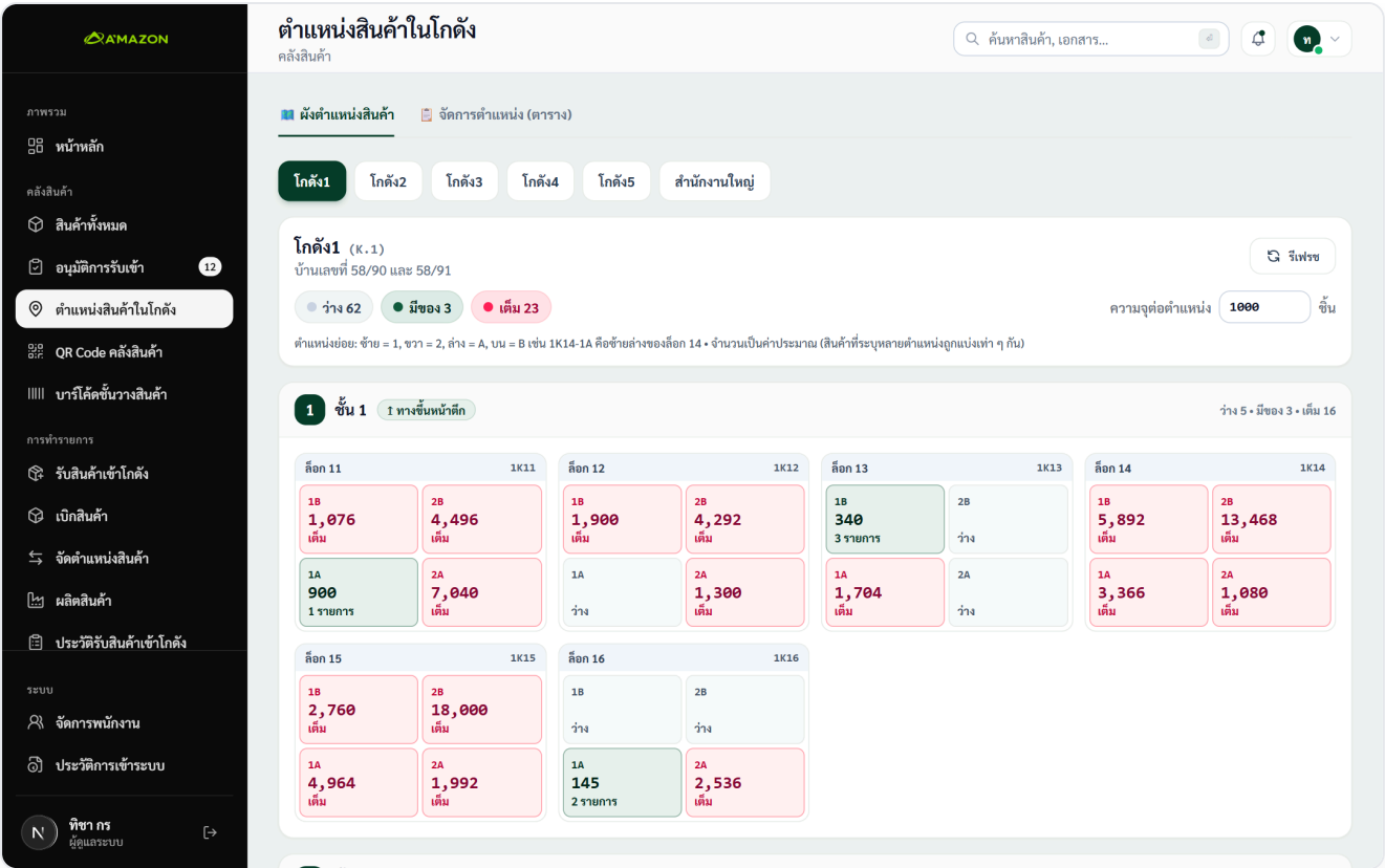
ภาพที่ 6.2: หน้าจอตรวจสอบแผนผังตำแหน่งชั้นวางสินค้าและจำนวนสต็อกประจำตำแหน่ง ( /locations )
