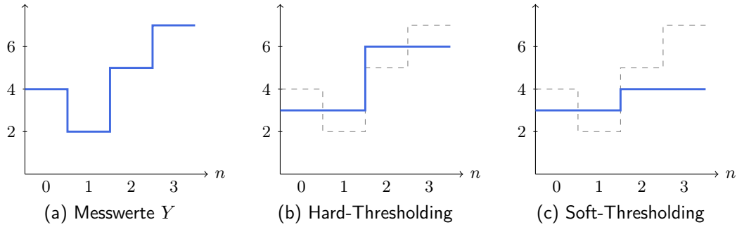
Abbildung 5.4.: Die Messwerte Y = (4, 2, 5, 7) aus Beispiel 5.8 (a) und die Schätzungen \hat{f} = (3, 3, 6, 6) nach Hard-Thresholding (b) und \hat{f} = (3, 3, 4, 4) nach Soft-Thresholding (c), jeweils mit T = 2 ; gestrichelt Y .
