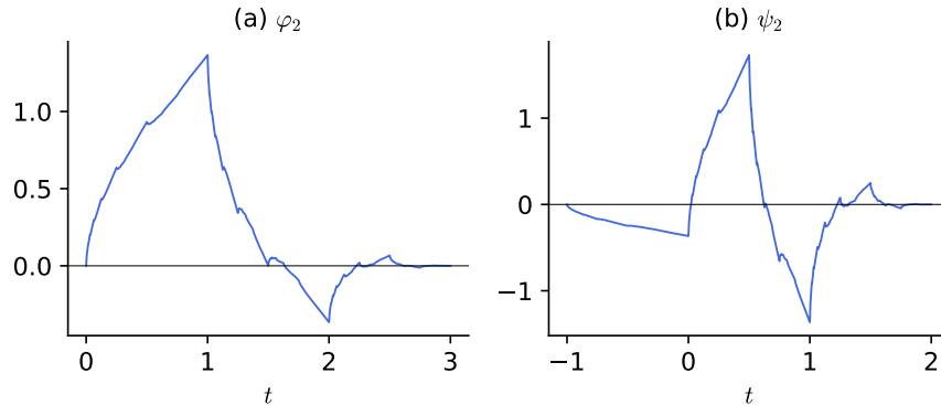
Abbildung 4.3.: Skalierungsfunktion \varphi_2 auf [0, 3] (a) und Wavelet \psi_2 auf [-1, 2] (b) zur Folge (4.6), berechnet durch Iteration der Skalierungsgleichung (4.1).
