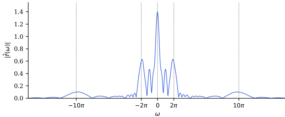
Abbildung 3.5.: Betragsspektrum |\hat{f}(\omega)| nach (3.5); gestrichelt die Stellen \pm 2\pi und \pm 10\pi .
