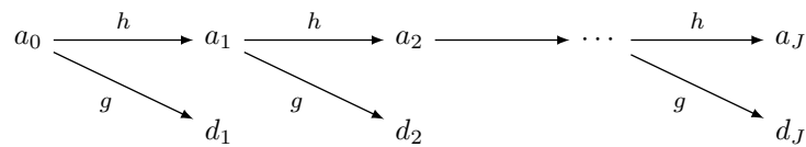
Abbildung 4.2.: Ablauf von Algorithmus 1, in Anlehnung an [Bla03, Kap. 5.4, (6)]; vgl. auch [LMR98, Abb. 2.8]. Jeder Pfeil ist ein Rechenschritt nach (4.11) mit dem Filter h bzw. g und halbiert die Anzahl der Werte. Nur die Approximationskoeffizienten werden weiter zerlegt.
