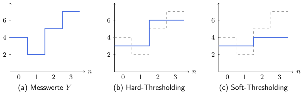
Abbildung 5.4.: Die Messwerte Y = (4, 2, 5, 7) aus Beispiel 5.8 (a) und die Schätzungen \hat{f} = (3, 3, 6, 6) nach Hard-Thresholding (b) und \hat{f} = (3, 3, 4, 4) nach Soft-Thresholding (c), jeweils mit T = 2 ; gestrichelt Y .
