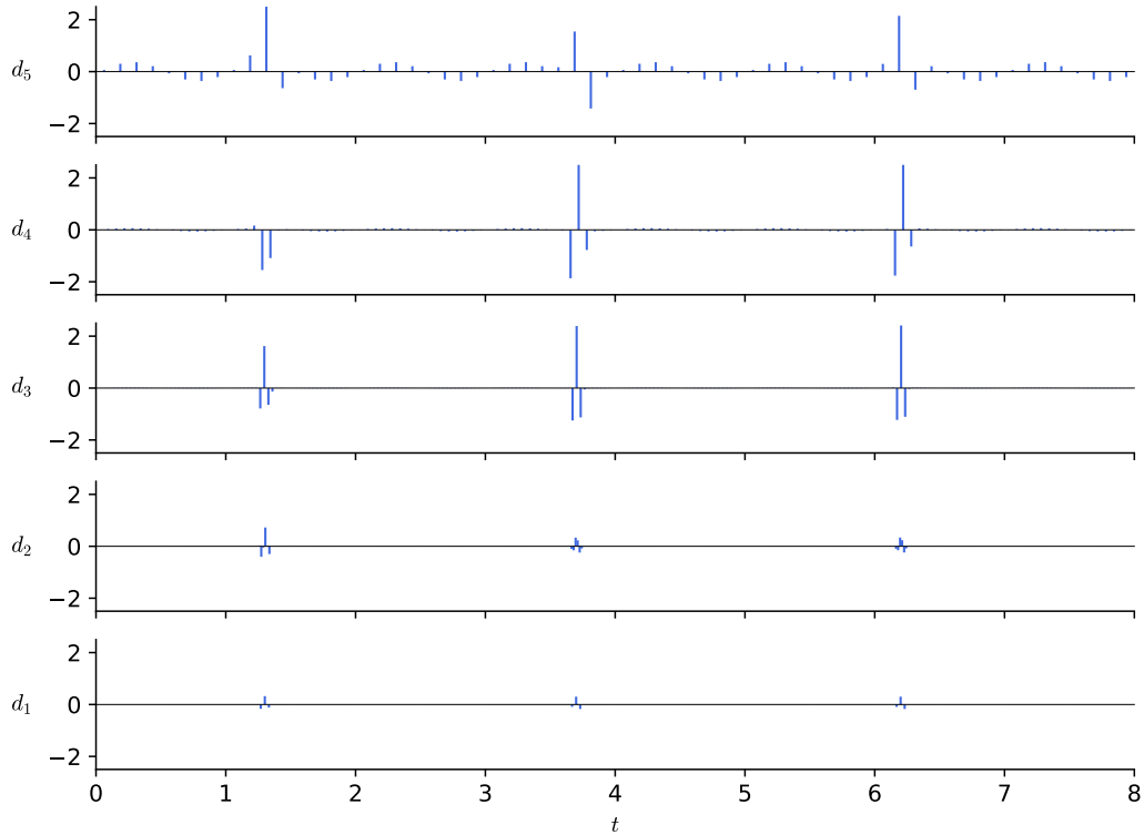
Abbildung 5.6.: Detailkoeffizienten d_5 (oben, grob) bis d_1 (unten, fein) des Testsignals f = u + s aus Beispiel 5.11, aufgetragen über der Zeit t ; sehr große Werte abgeschnitten.
