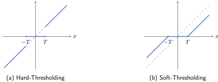
Abbildung 5.3.: Die Funktionen \rho_T^H (a) und \rho_T^S (b); gestrichelt die Identität.
