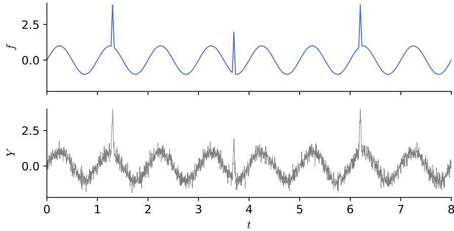
Abbildung 5.5.: Das Testsignal f = u + s aus Beispiel 5.11 (oben) und die Beobachtung Y = f + 0,3 Z (unten), N = 2048 (Code in Anhang B.4).
