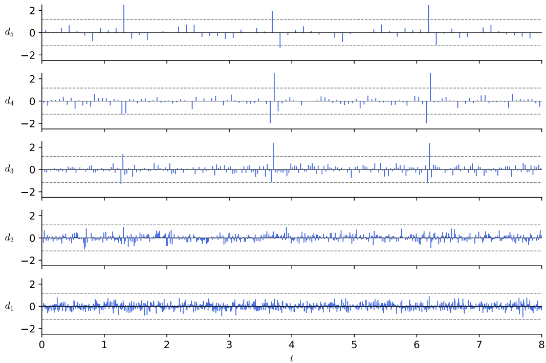
Abbildung 5.7.: Detailkoeffizienten d_5 (oben) bis d_1 (unten) der Messwerte Y = f + 0,3 Z aus Beispiel 5.13, im selben Maßstab wie Abbildung 5.6; gestrichelt die Schwelle \pm T = \pm 1,17 .
