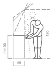
b./ ALACSONY TÁROLÓ
