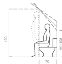
h./ WC BERENDEZÉS HASZNÁLATA
