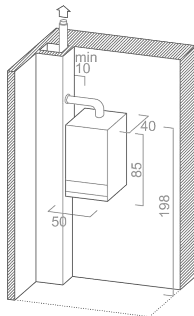
b./ szerelt kéményhez csatlakoztatva
