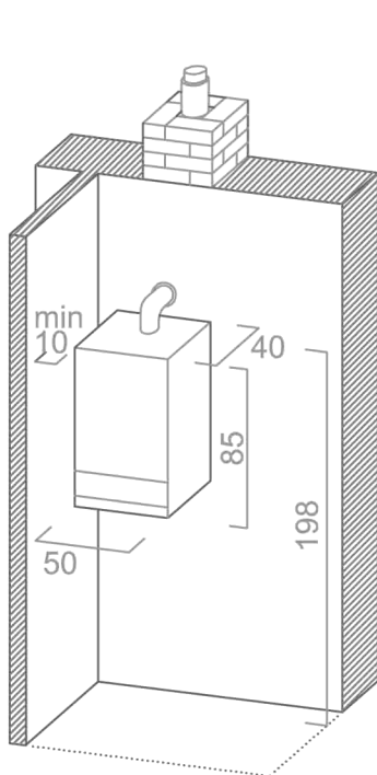
a./ falazott, bélelt kéményhez csatlakoztatva
