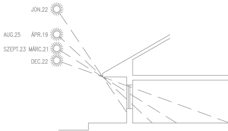
DÉLI HOMLOKZAT ÁRNYÉKOLÁSA VÍZSZINTES ÁRNYÉKOLÓ SÍKKAL
