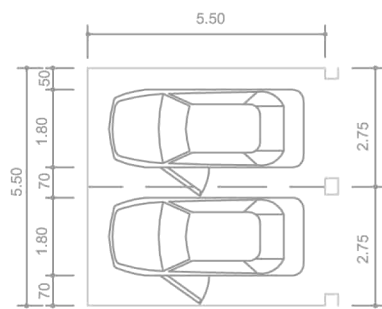
IKER GÉPKOCSITÁROLÓ
