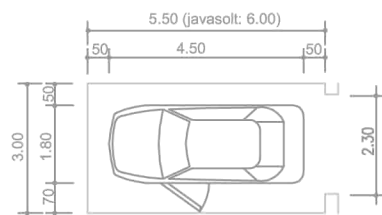
ZÁRT GÉPKOCSITÁROLÓ
