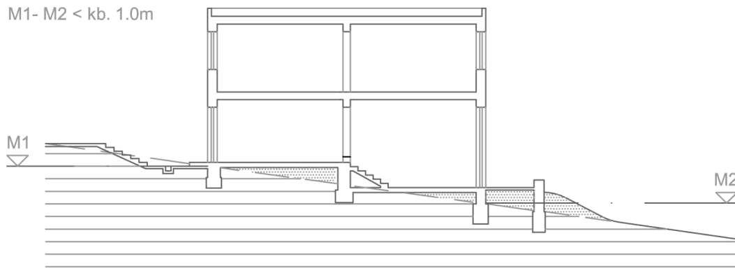
a./ LEJTÉS KÖVETÉSE A BELMAGASSÁG VÁLTOZTATÁSÁVAL
