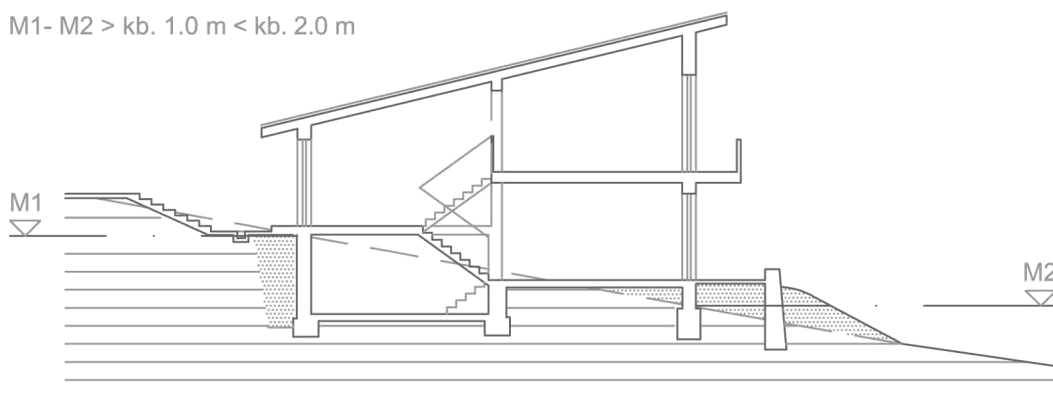
b./ LEJTÉS KÖVETÉSE FÉLSZINT-ELTOLÁSSAL
