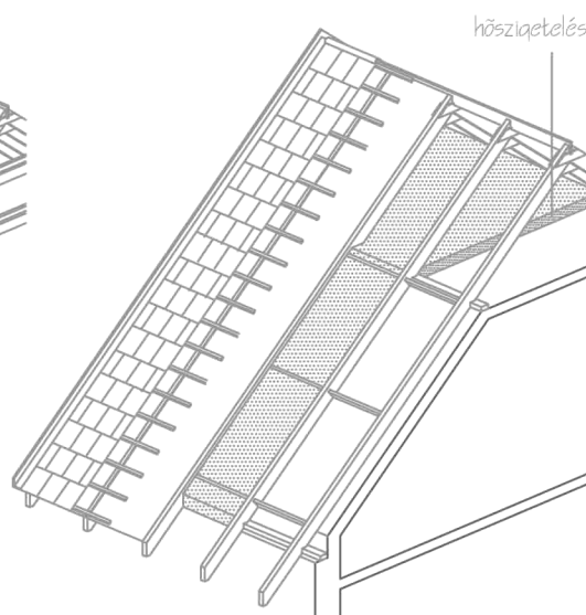
c./ vasbeton födémen ("koporsófödém") fekvő szaruzat
