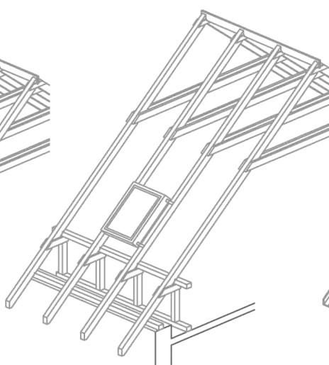
b./ fekvő tetőablak elhelyezése
