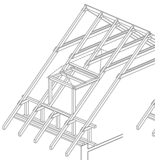
a./ álló tetőablak ácsolata
