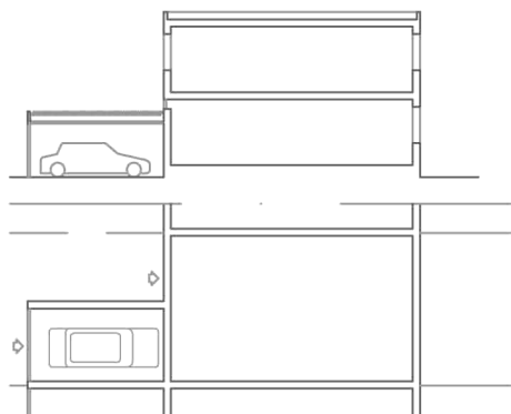
b./ Gépkocsitároló az egység előtt
