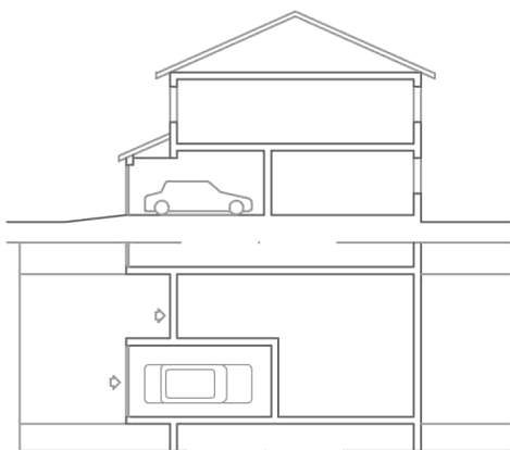
a./ Gépkocsitároló keskeny egységen belül
