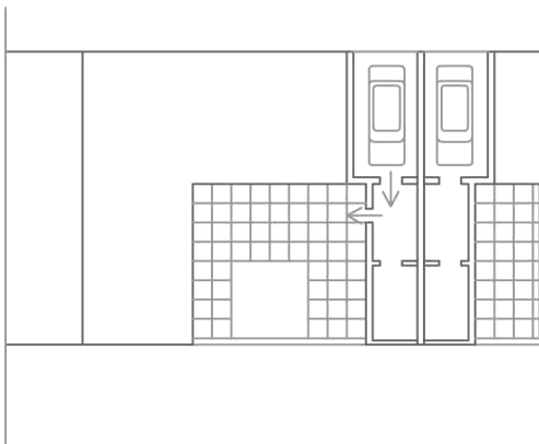
e./ gépkocsitároló a kiegészítő helyiségekhez kapcsolódik
