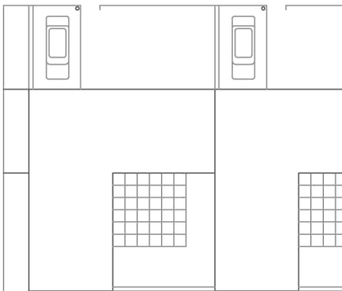
c./ fedett, nyitott gépkocsibeálló az előkertben
