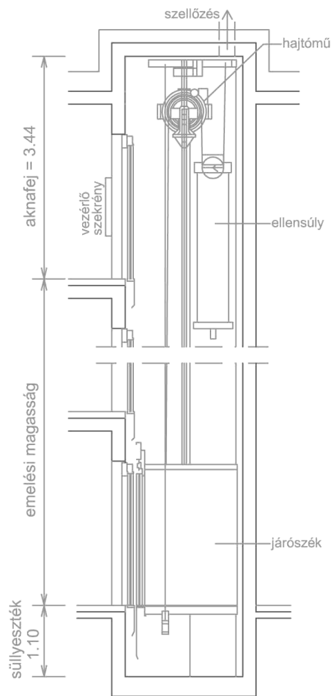
FELVONÓAKNA METSZETE
