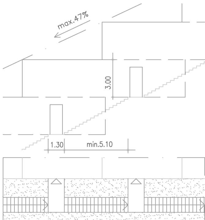
A./ EGYENES VONALÚ, EGYKARÚ TEREPLÉPCSŐ
