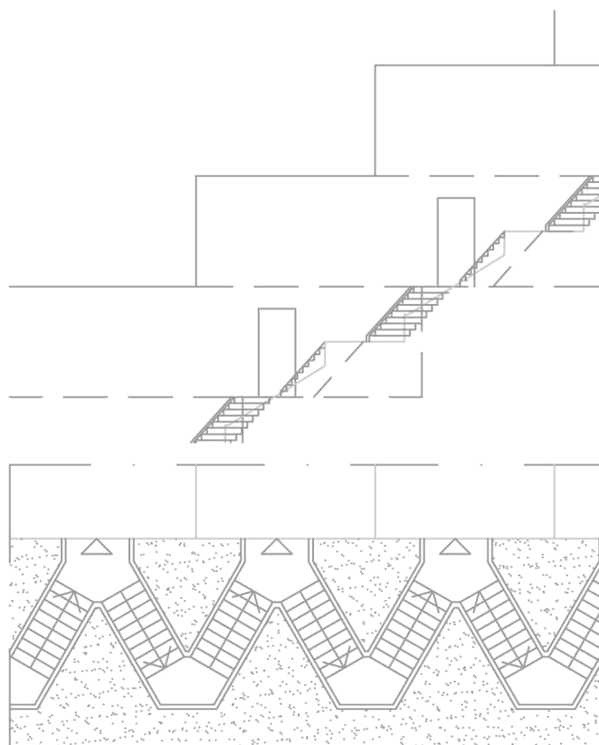
B./ KÉTKARÚ TEREPLÉPCSŐ
