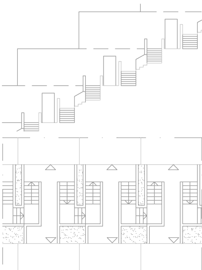
C./ HÁROMKARÚ TEREPLÉPCSŐ, KÉTSÁVOS FELTÁRÁS
