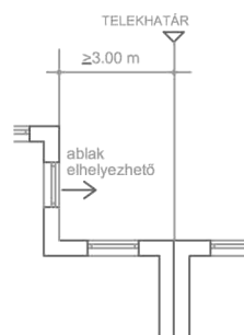
e./ Kiugró épületrész a telekhatártól távolabb
