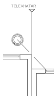
a./ Részleges tűzfaltakarás (Szomszéd benapozása!)
