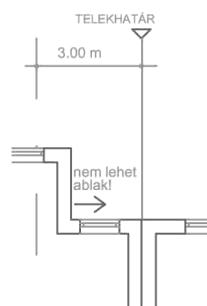
d./ Kiugró épületrész a telekhatár közelében
