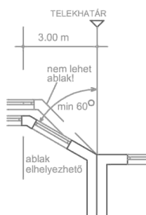
c./ Ablak a ferde szögben csatlakozó homlokzati falon
