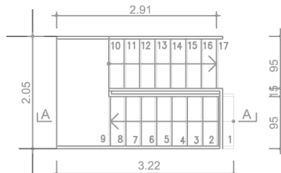
Kétkarú lépcső
