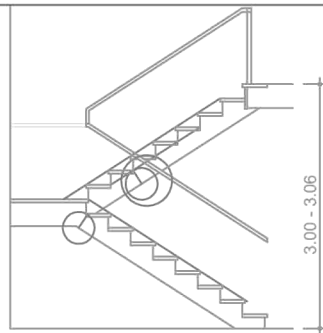
A-A metszet
