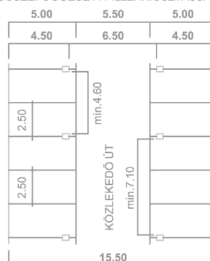
A KÖZLEKEDŐ ÚT SZÉLESSÉGÉNEK ÖSSZEFÜGGÉSE A PILLÉRKIOSZTÁSSAL
