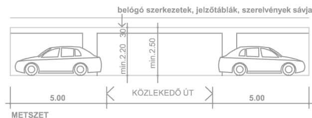
A KÖZLEKEDŐ ÚT SZÉLESSÉGÉNEK ÖSSZEFÜGGÉSE A PILLÉRKIOSZTÁSSAL
