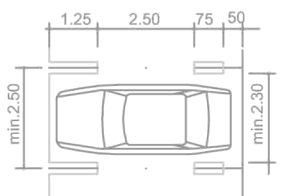
A GÉPKOCSI HELYZETE KÜLÖNBÖZŐ PILLÉRKÖZÖKBEN
