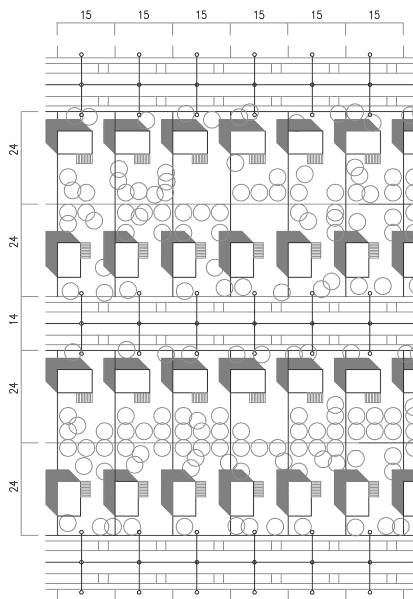
a./ "HAGYOMÁNYOS" APRÓTELKES ELRENDEZÉS
