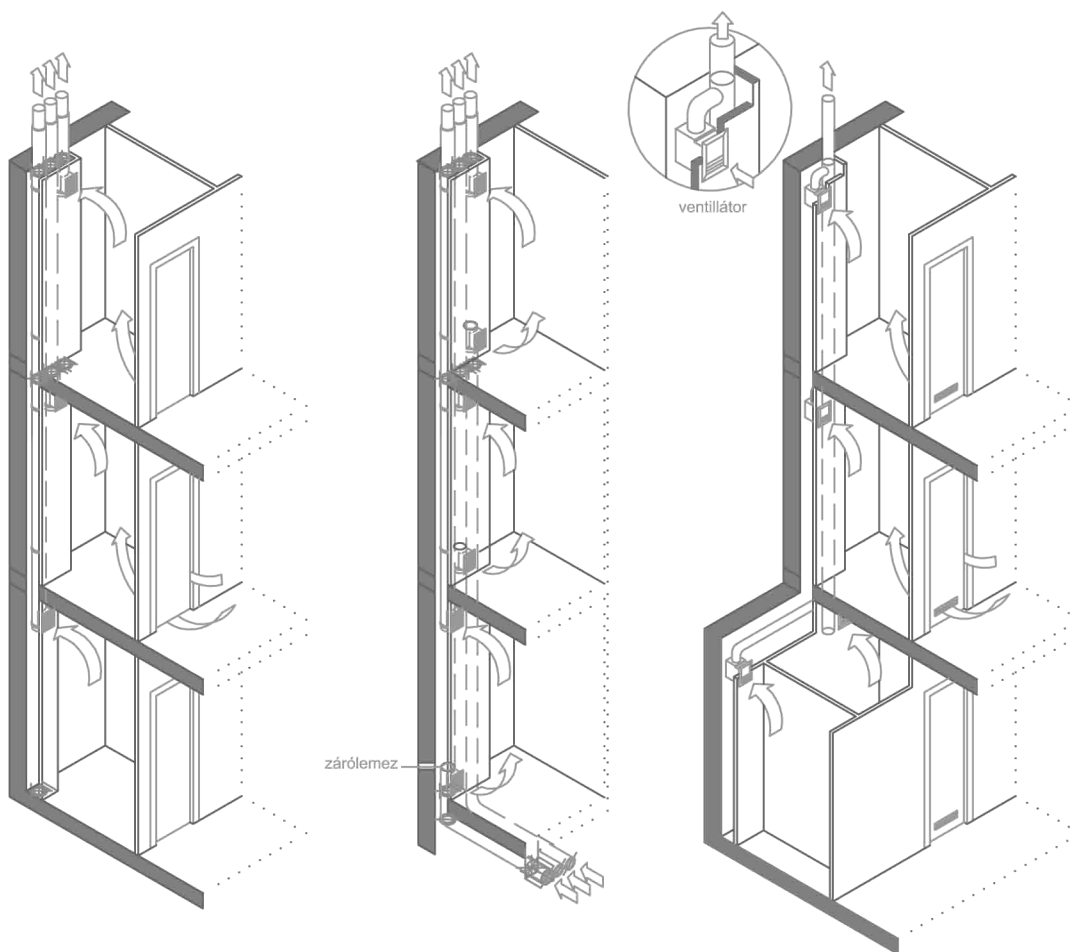
a./ GRAVITÁCIÓS SZELLŐZÉS FRISSLEVEGŐ-UTÁNPÓTLÁS NÉLKÜL
