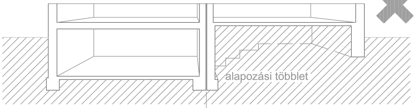
c./ Csak egyik épület alápincézve: KERÜLENDŐ!
