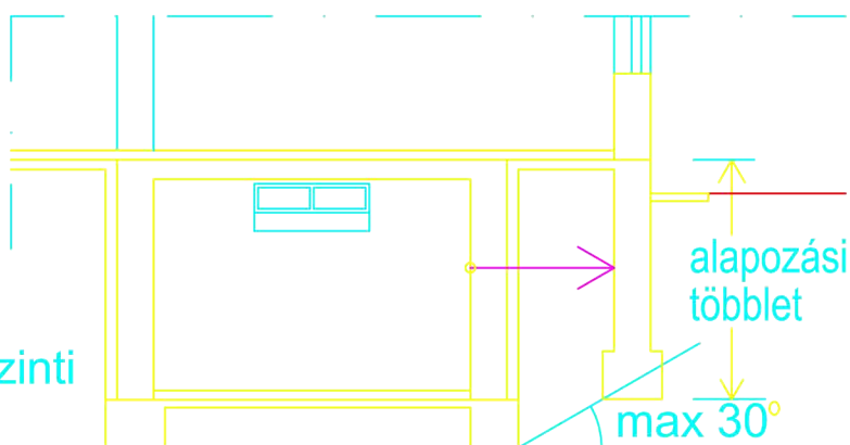
c./ RÉSZLEGES ALÁPINCÉZÉS HELYTELEN MÓDJA
