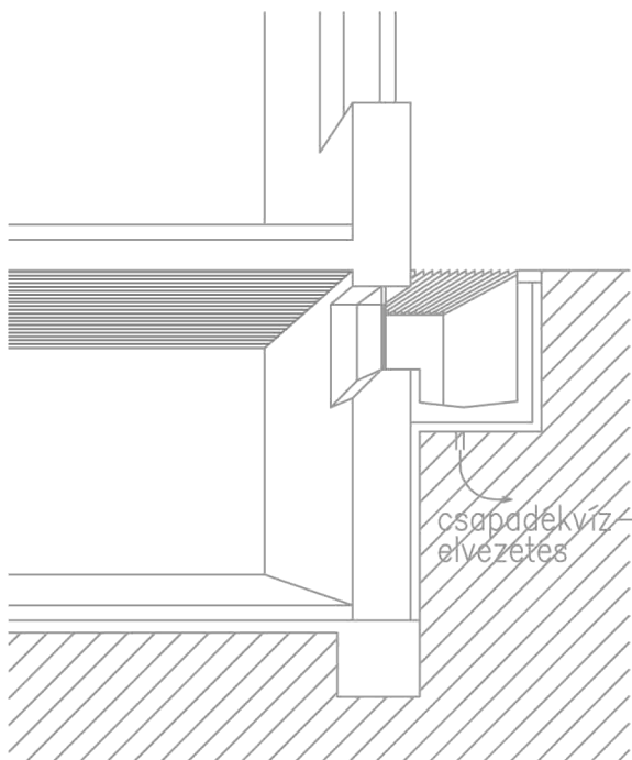
PERSPEKTIVIKUS METSZET
