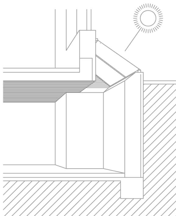
PERSPEKTIVIKUS METSZET
