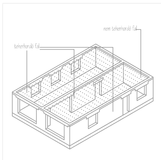
b./ HOSSZFALAS ELRENDEZÉS
