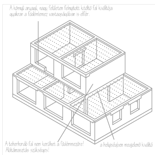
f./ RÉSZBEN KÉTSZINTES
