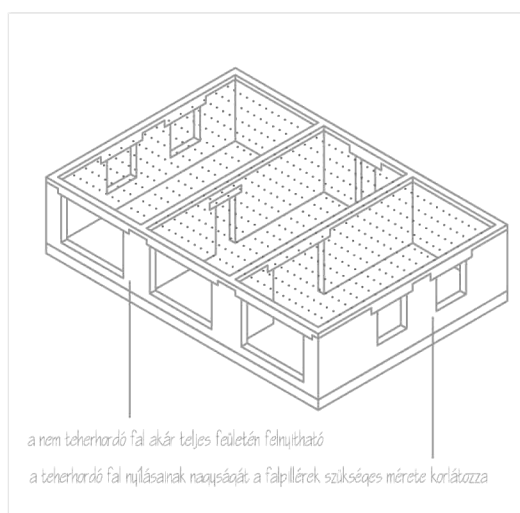
c./ HARÁNTFALAS ELRENDEZÉS
