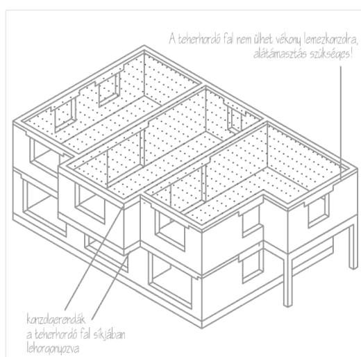
e./ EMELETI KONTÚR NAGYOBB
