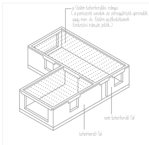
a./ EGYMENETES ELRENDEZÉS
