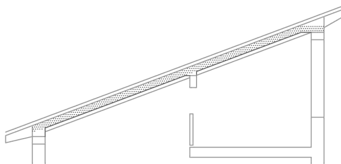
j./ fa-zárófödémrel egyesített mérsékelt hajlásszögű félnyereg-tető
