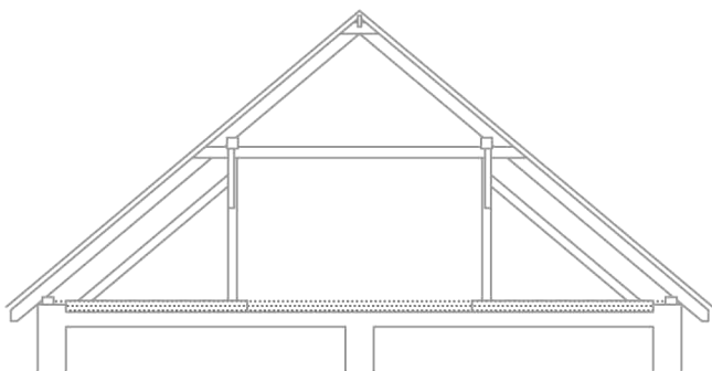
e./ két állószékes, hagyományos fedélszék
