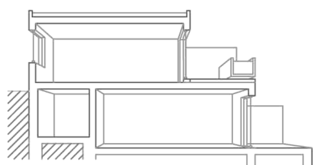
l./ Teraszház-jellegű kétszintes sorház lejtős terepen
