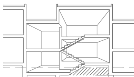
k./ Hossztengely irányában szinteltolós sorház
