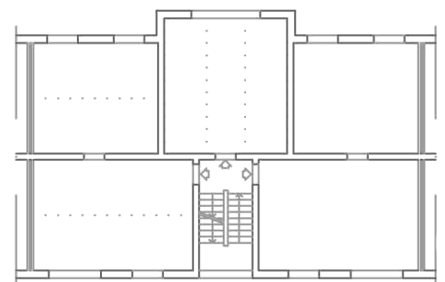
haránt- és hosszafalás
